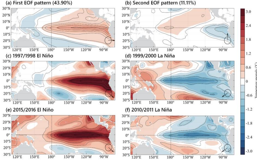
Figure 12: Distribution of (a) first and (b) second EOF patterns of observed SSTA, and spatial patterns of SSTA in (c) 1997/1998 El Niño, (d) 1999/2000 La Niña, (e) 2015/2016 El Niño, and (f) 2010/2011 La Niña.
