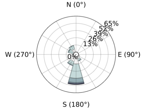
(d) NZWAVE-ST6
