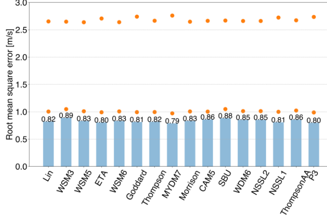
(d) Model RMSE [m/s]
