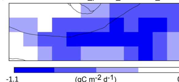
(d) GPP RMSD: ISBA_pheno_irr – ISBA_ref
