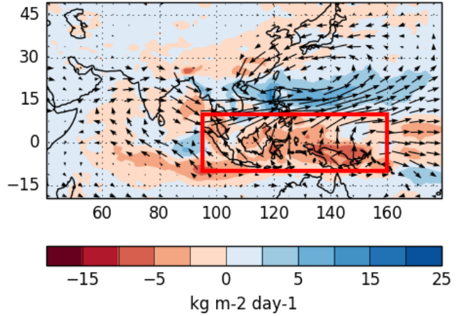
(d) Control minus nudged Maritime Continent JJA clim difference \rightarrow 2 \text{ m/s}
