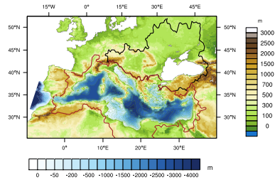
(d) MESONH-Symphonie
