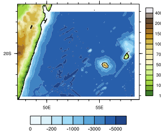
(e) MESONH-NEMO
