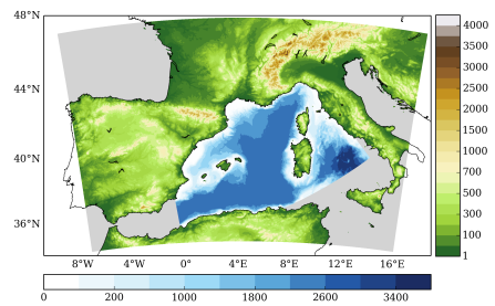
(d) MESONH-Symphonie
