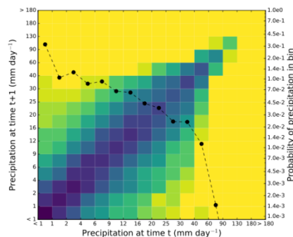
f. N512@N48 EQ region
