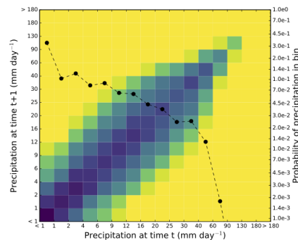
c. N512@N48 EQ region
