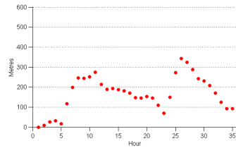
(d) Contour, 10m current
