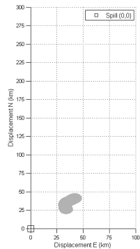
(d) CranSLIK, hr 277, 0m current
