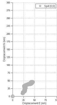
(d) CranSLIK, hr 240, 0m current
