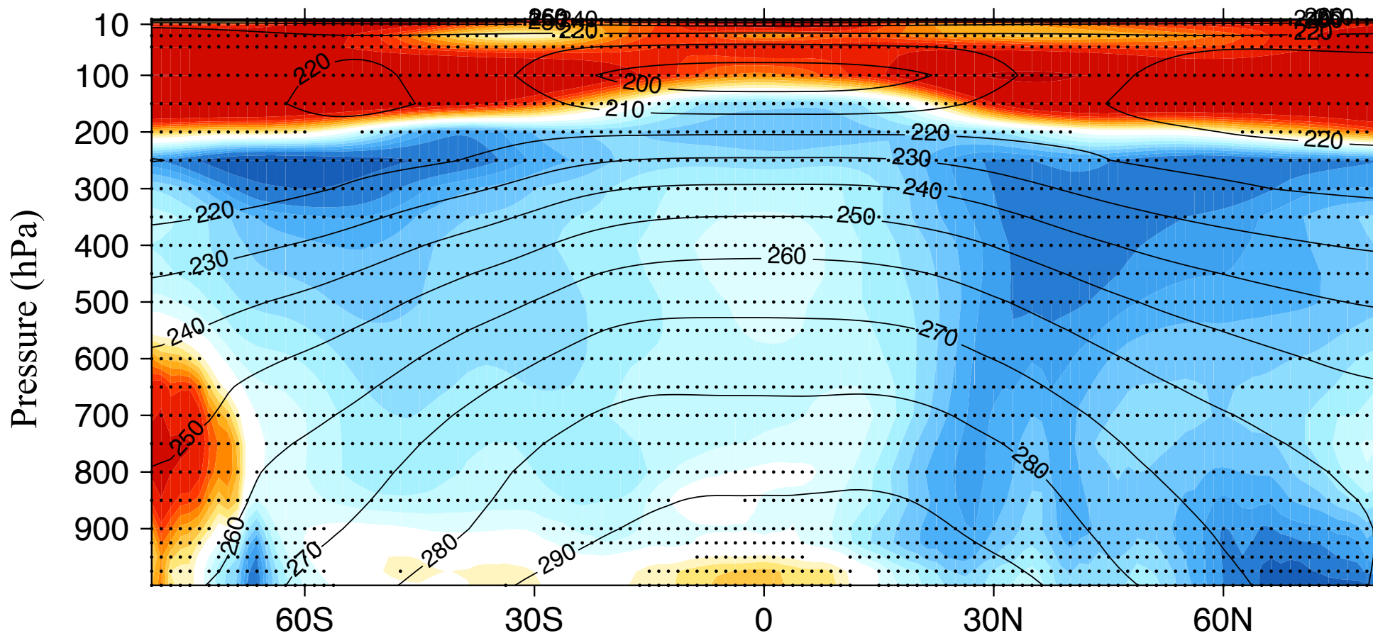
(c) A-K31 (contours) ; A-K31 minus A-K31 (shading)
