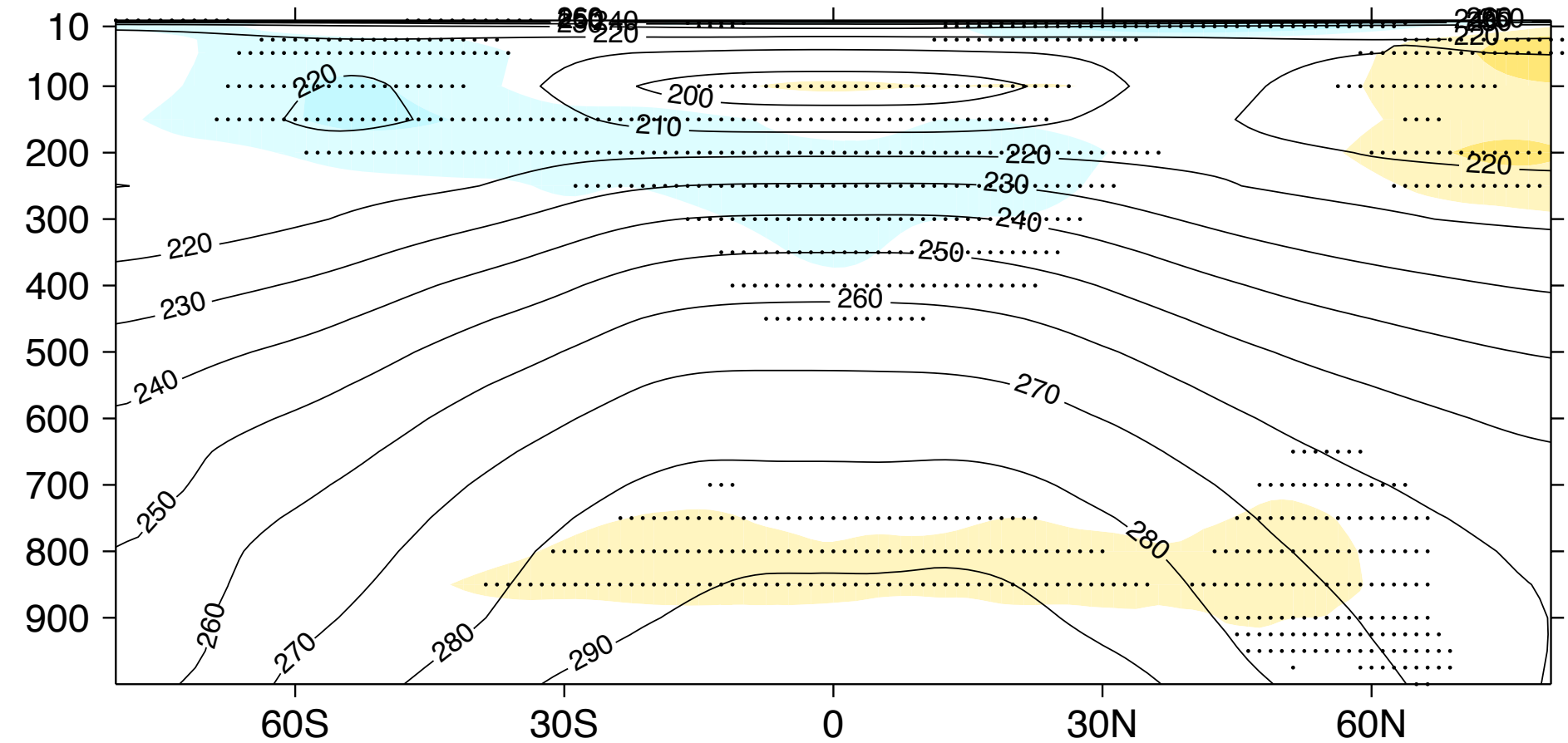
(d) K-O (contours) ; K-O minus A-K31 (shading)
