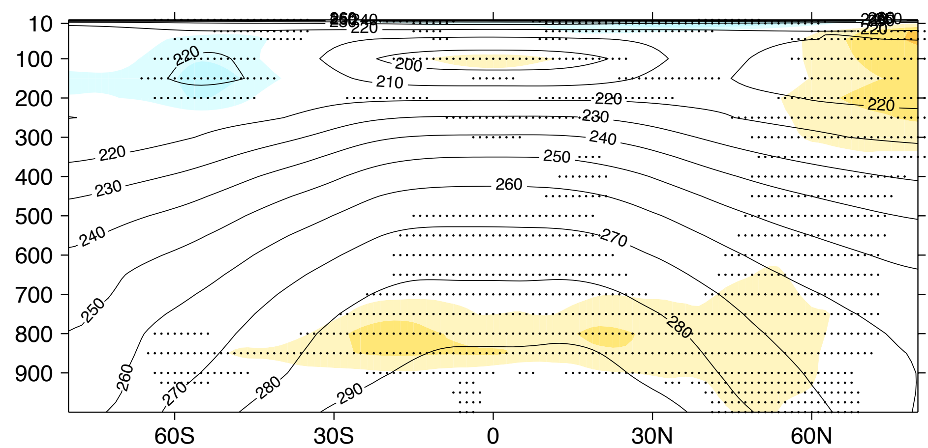
(d) K-O (contours) ; K-O minus A-K31 (shading)
