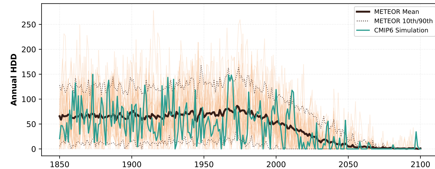
Cairo - HDD
