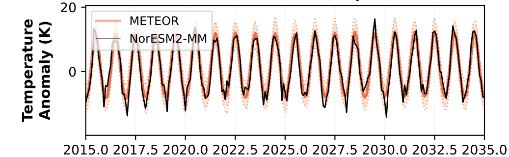
Delhi (28.6°, 77.2°) - Temperature
