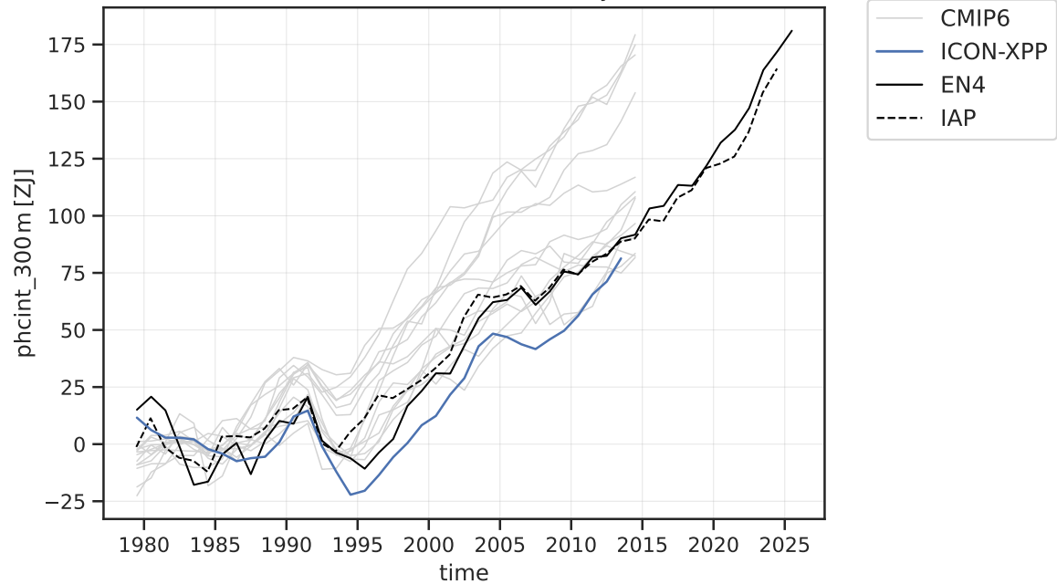
Global Ocean Heat Content Anomaly (0-300 m)
