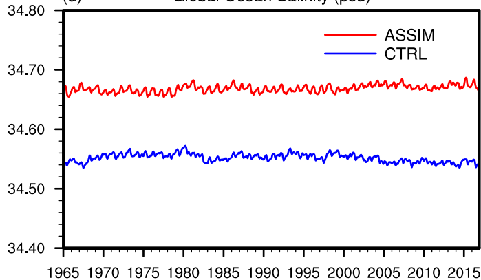
(d) Global Ocean Salinity (psu)
