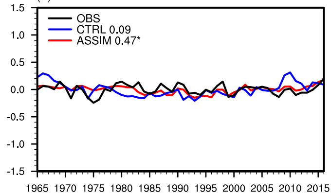
(d) Ocean detrended T2m
