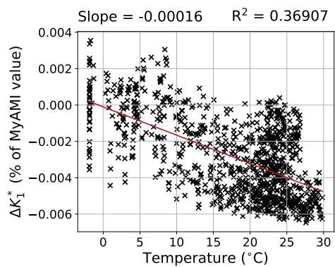
g) K_1^*
