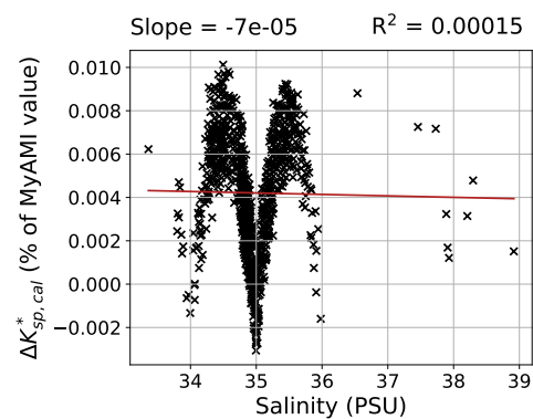
f) K_{sp,cal}^*
