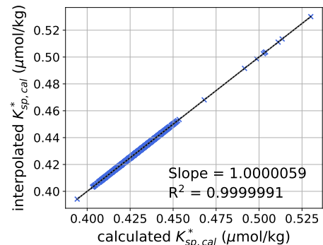
f) K_{sp,cal}^*
