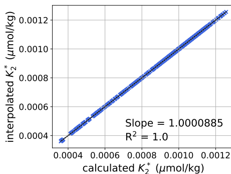
e) K_2^*
