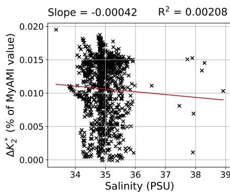
e) K_2^*
