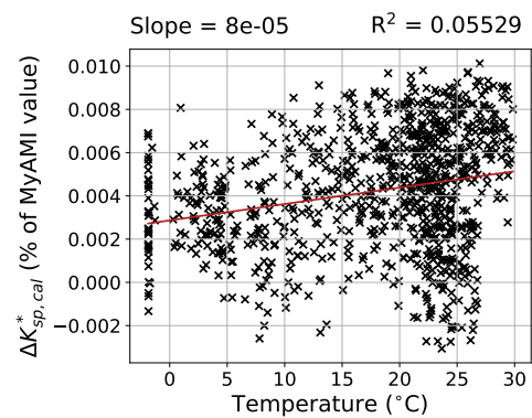
i) K_{sp,cal}^*
