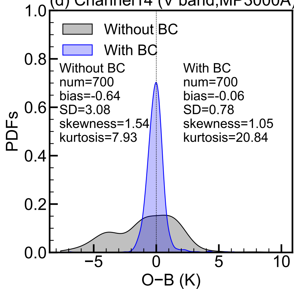
(d) Channel14 (V band,MP3000A)
