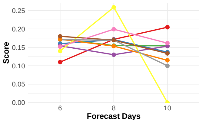
(b) SEDI
