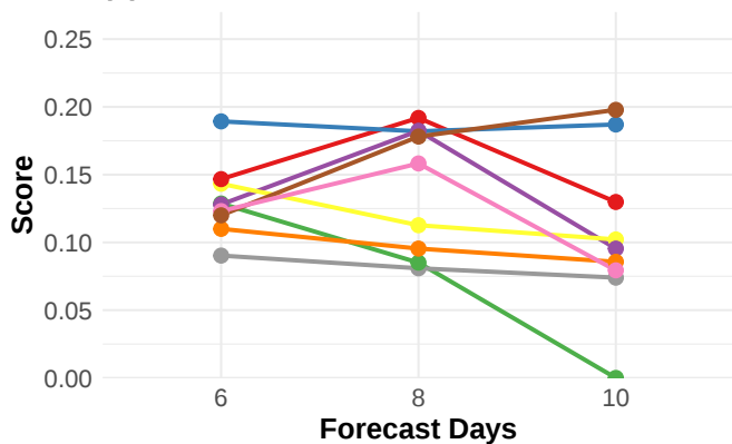
(d) SEDI
