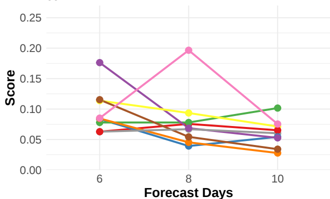
(f) SEDI
