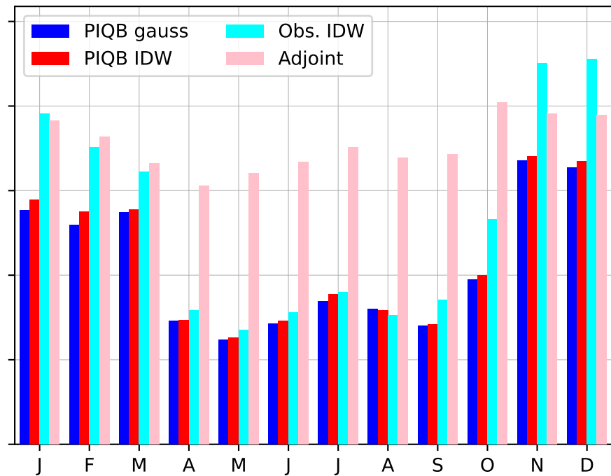
CAMx
