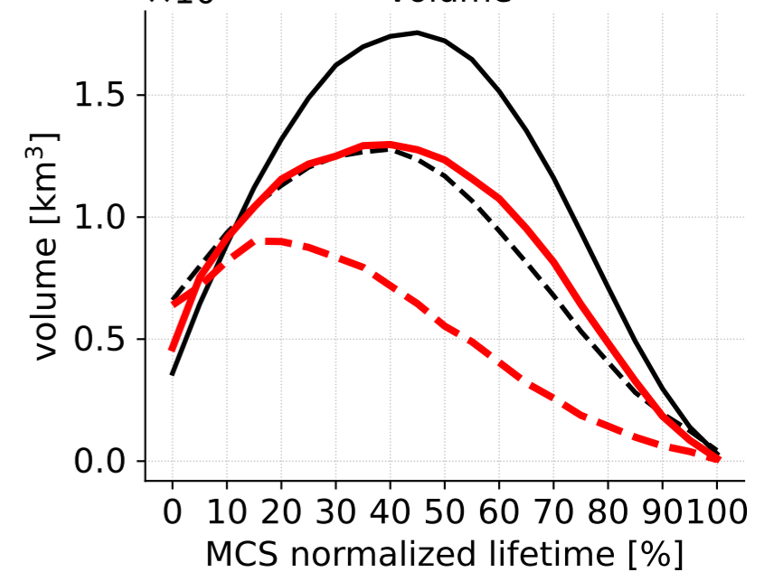
l) land tropics volume
