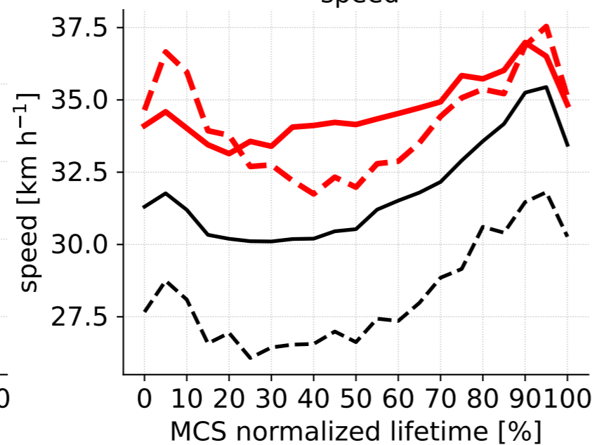
g) ocean tropics speed
