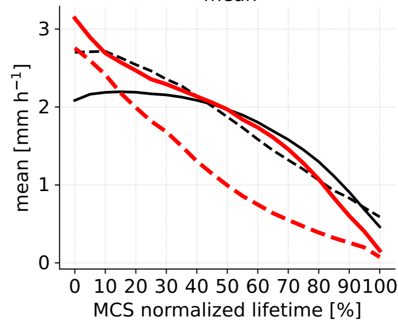
j) land tropics mean
