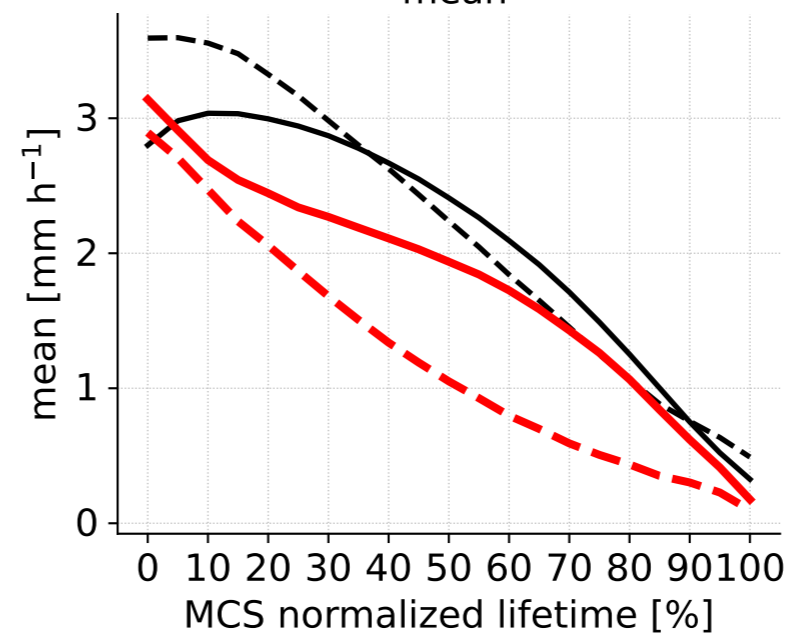
i) ocean tropics mean
