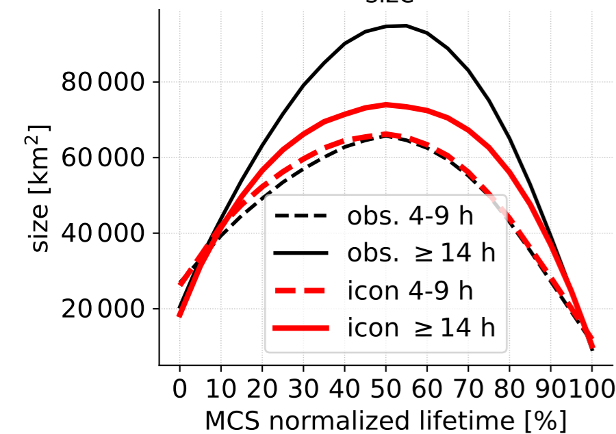
e) ocean tropics size
