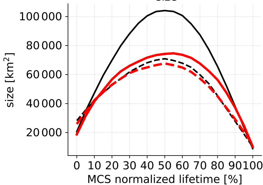
f) land tropics size
