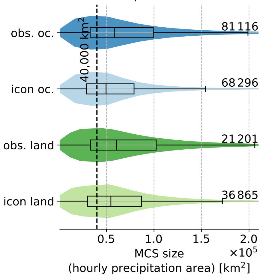
e) ocean tropics size
