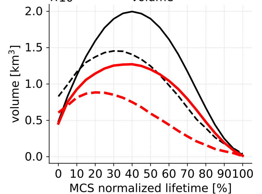
k) ocean tropics volume
