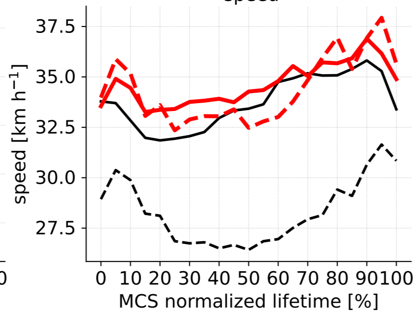
h) land tropics speed
