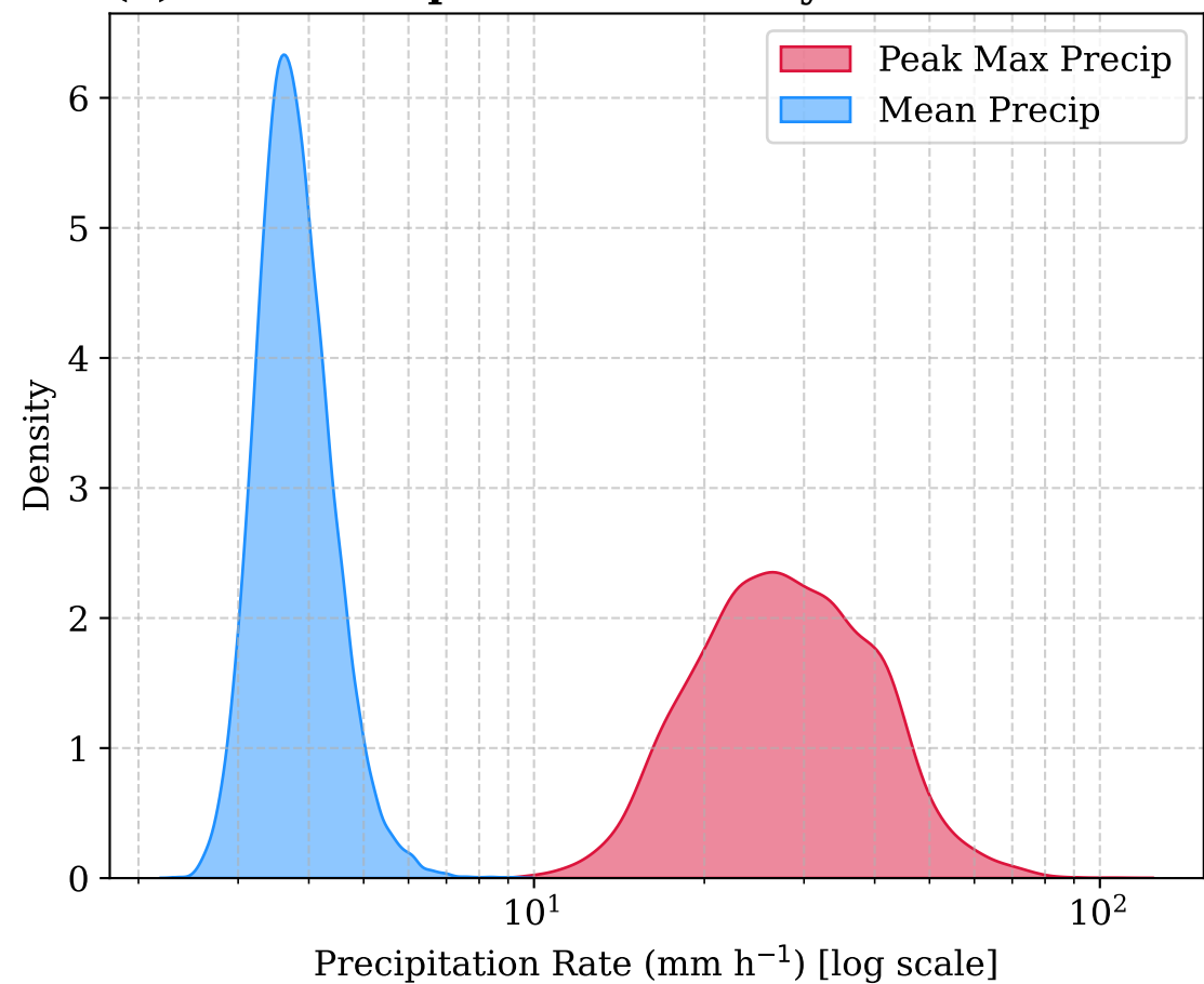
(d) MCS Precipitation Intensity
