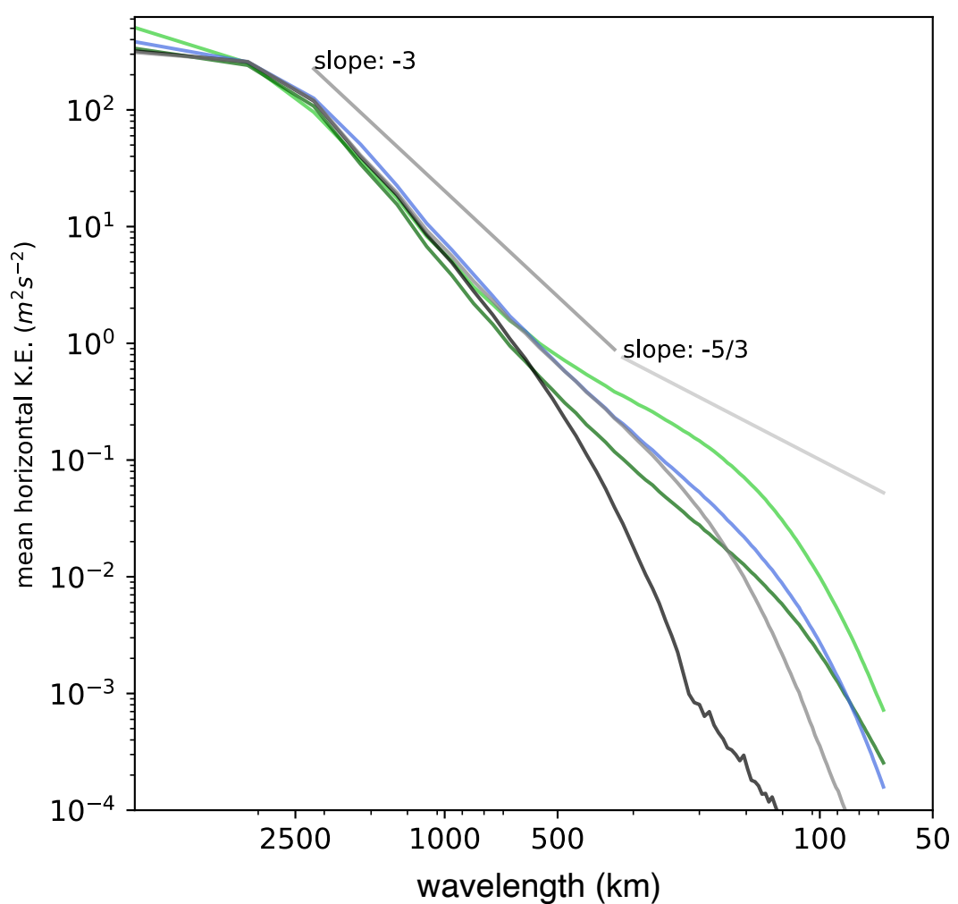
(d) Horizontal winds at 200 hPa
