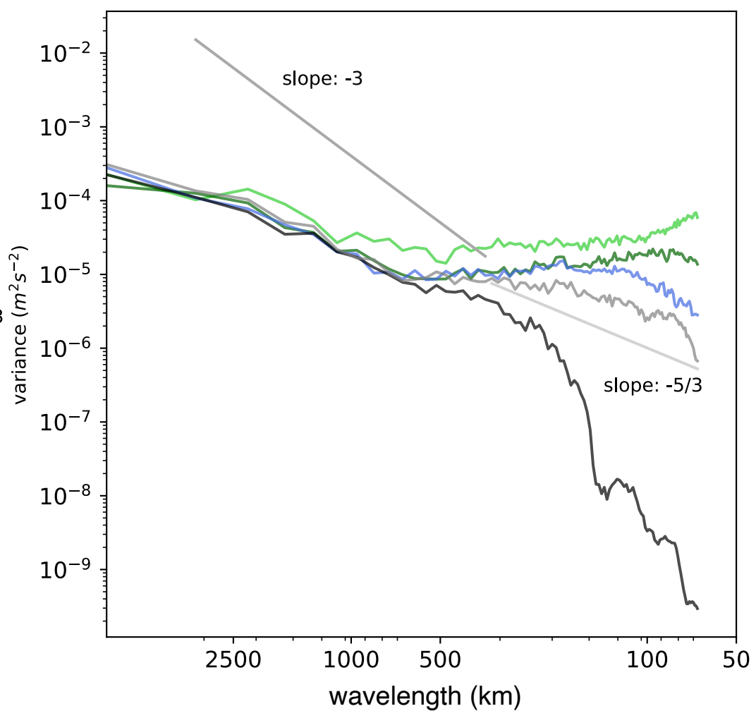
(d) Horizontal winds at 200 hPa
