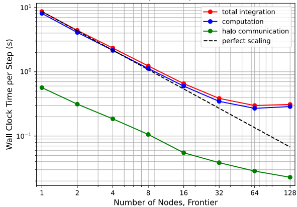
MPAS-Ocean GPU, Frontier, 1024x1024x96
