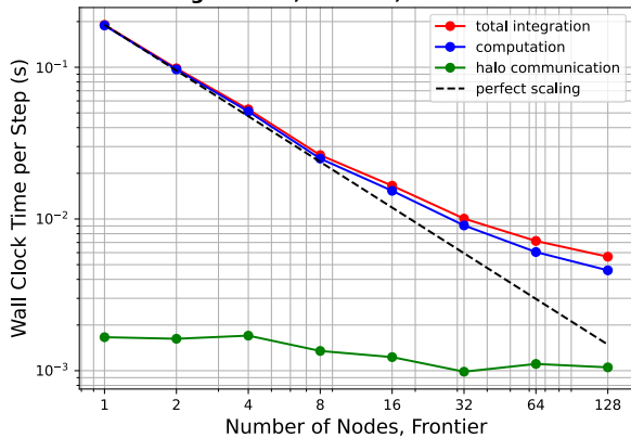
Omega-0 GPU, Frontier, 1024x1024x96
