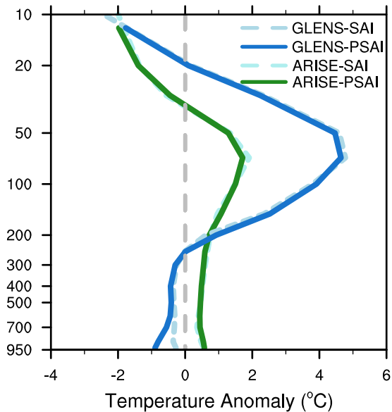
b) ARISE/GLENS-SAI versus PSAI
