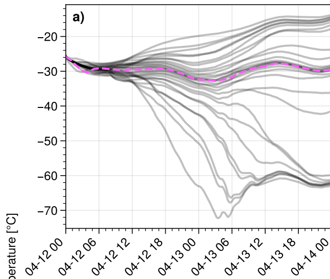
OIFS 40r1 – NEMO 3.6
