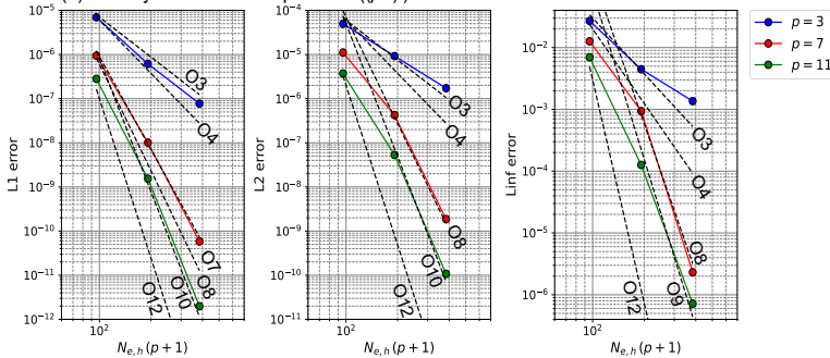
(d) Density x Potential temperature ( \rho\theta' )
