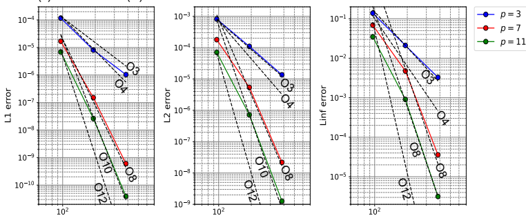
(d) Density x Potential temperature ( \rho\theta' )
