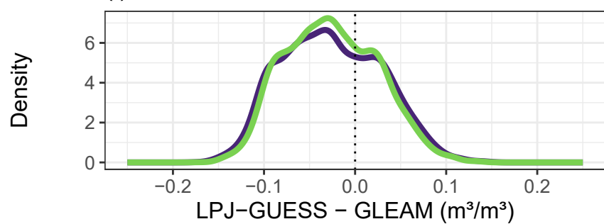
(i) Root-zone SM
