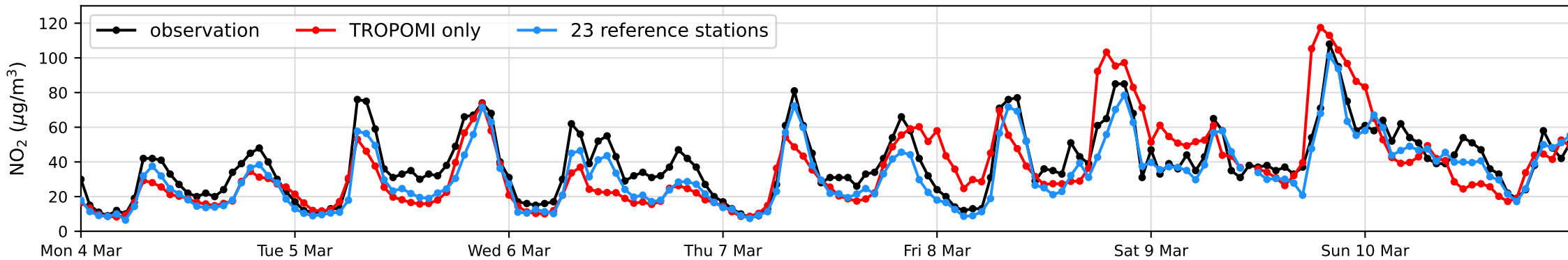
NO 2 concentrations at Parque del Retiro (ES1939), urban background
