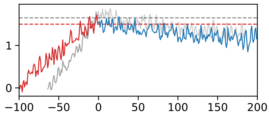
MPI-ESM1-2-LR
