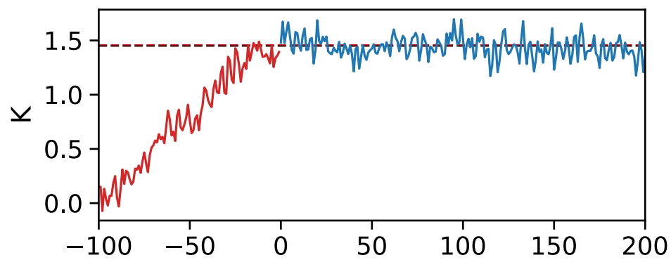
GFDL-ESM4
