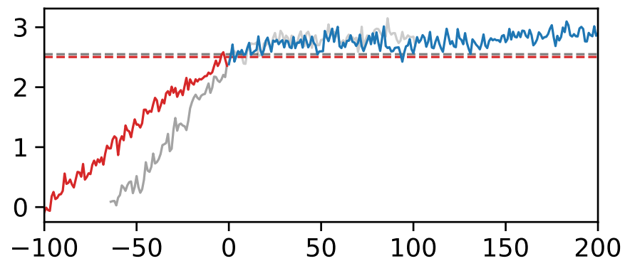
UKESM
