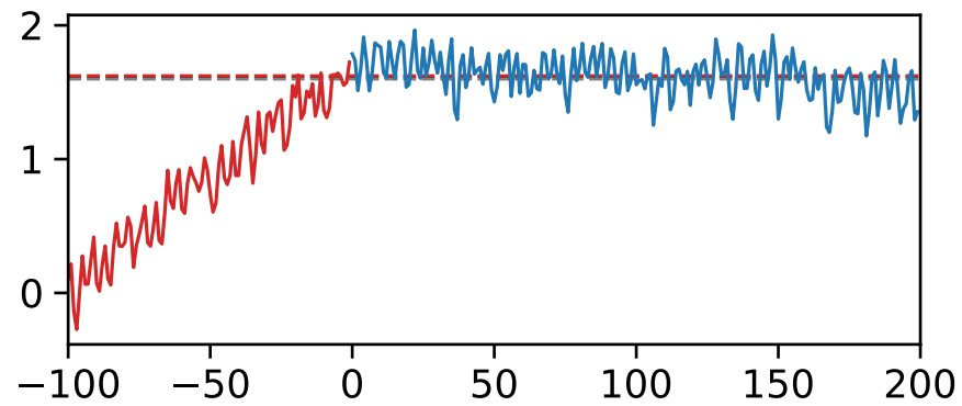
GISS
