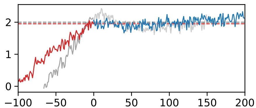
CESM2
