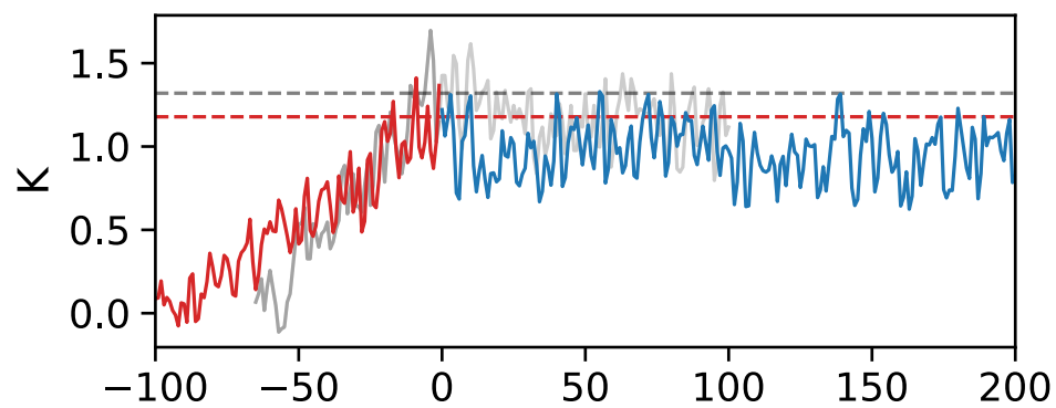
NorESM2-LM
