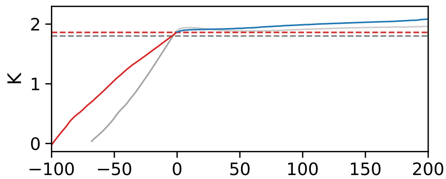
UVic-ESCM-2-10
