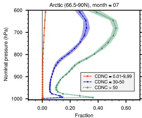
(d) Fraction of grid box with cloud base
