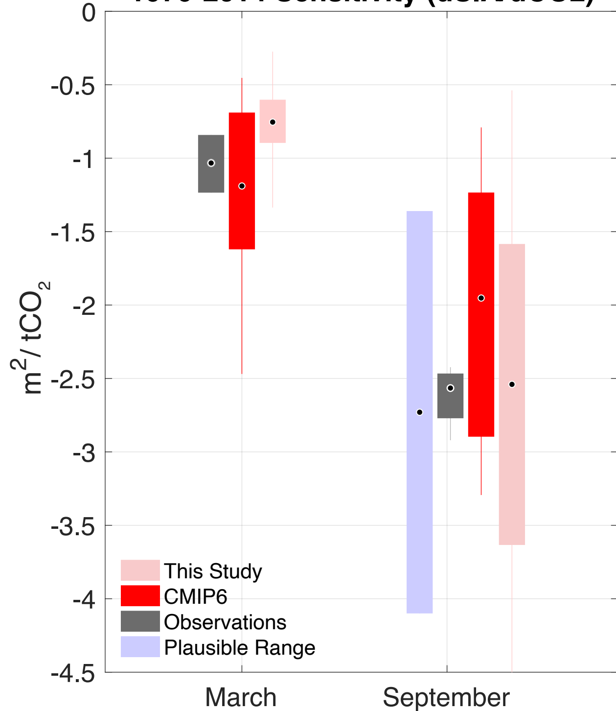
1979-2014 Sensitivity (dSIA/dCO2)
