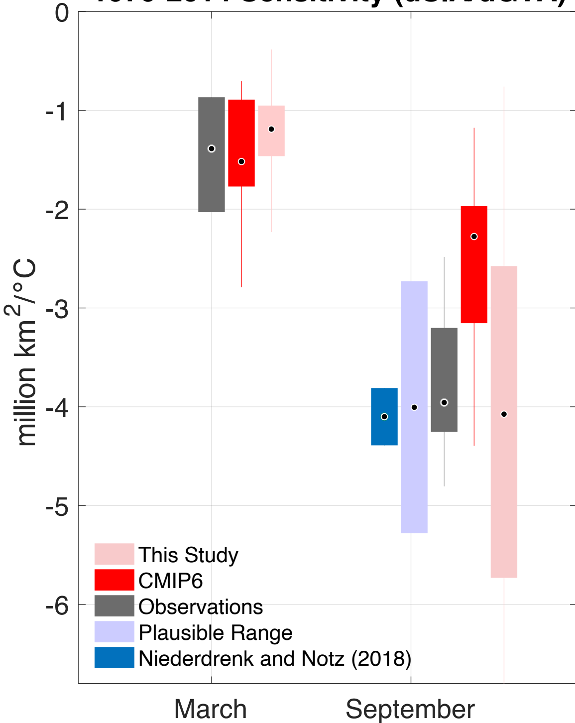
1979-2014 Sensitivity (dSIA/dGTA)
