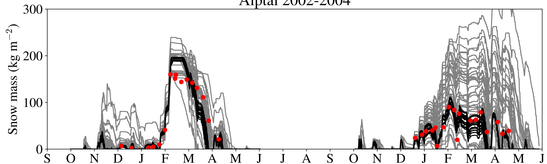
BERMS OJP 2002-2004
