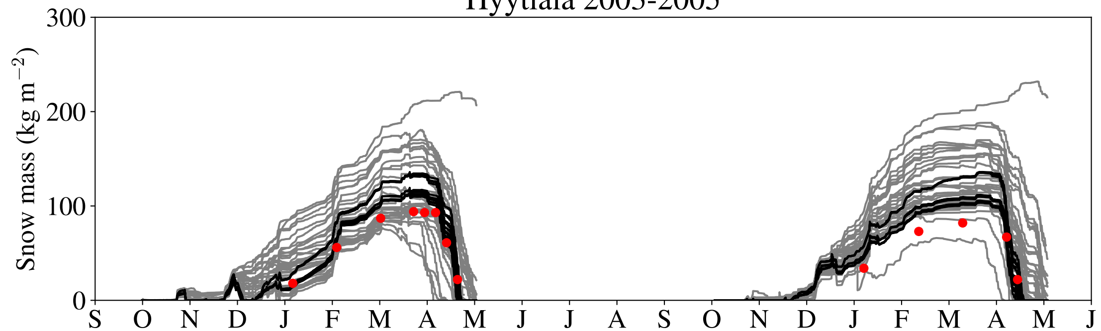
Hyytiala 2003-2005
