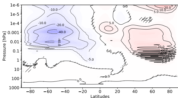
(d) \Delta \text{NGWD}
