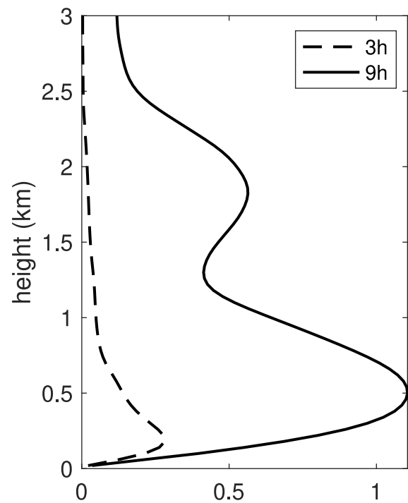
(a) \langle w'w' \rangle ( \text{m}^2\text{s}^{-2} )
