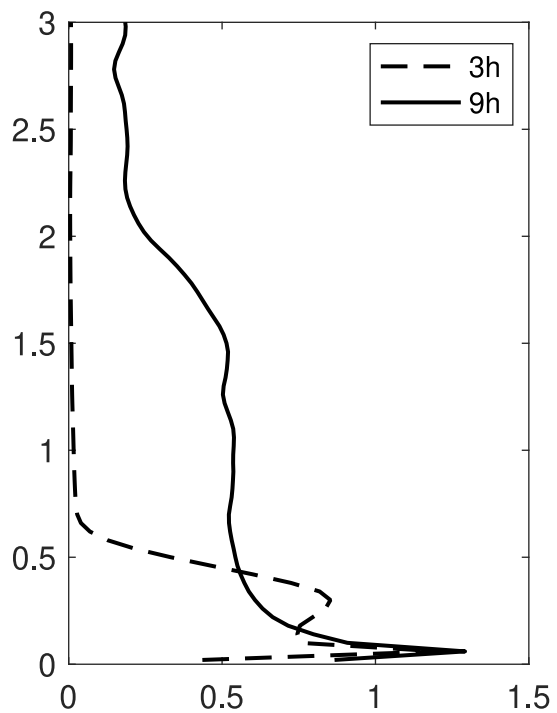
(b) \langle u'u' \rangle ( \text{m}^2\text{s}^{-2} )
