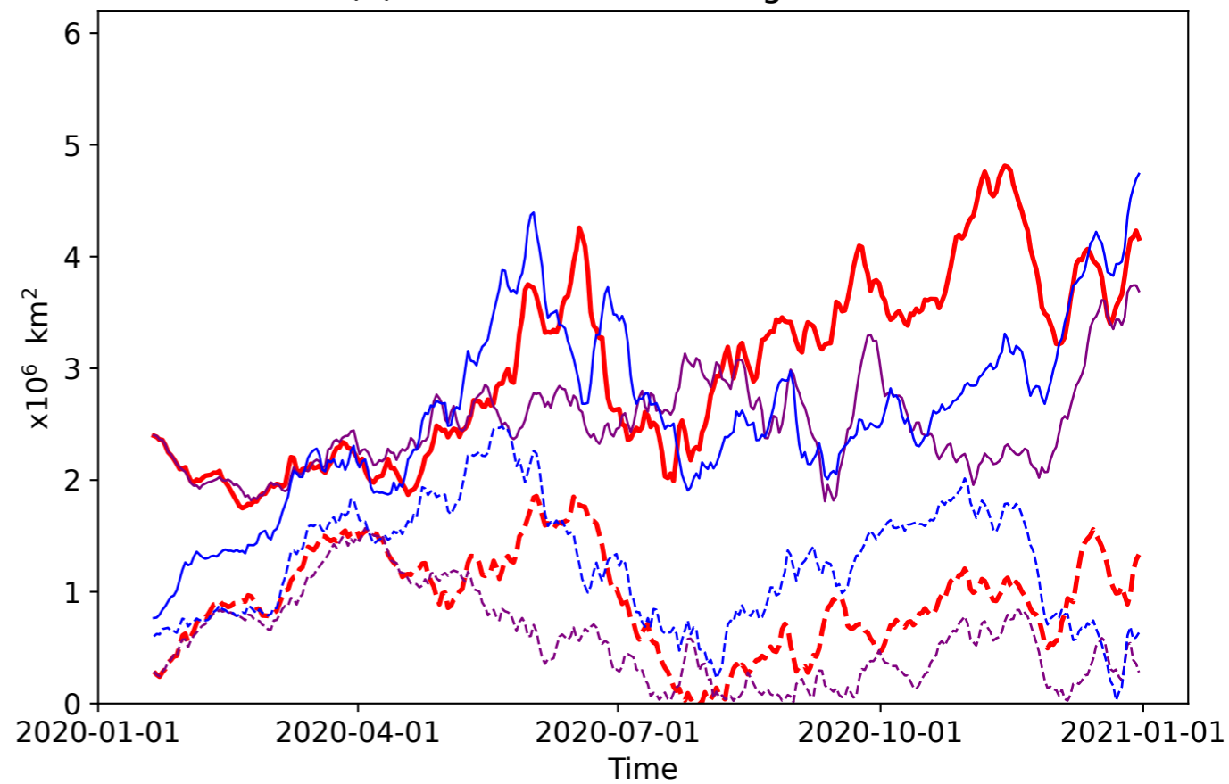
(d) Antarctic Sea Ice Extent
