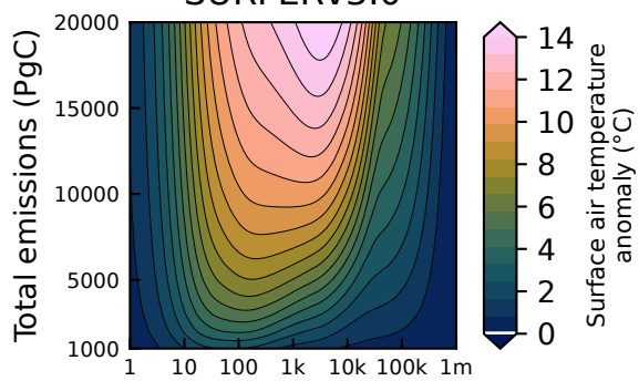
SURFERV3.0
