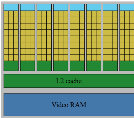
GPU
