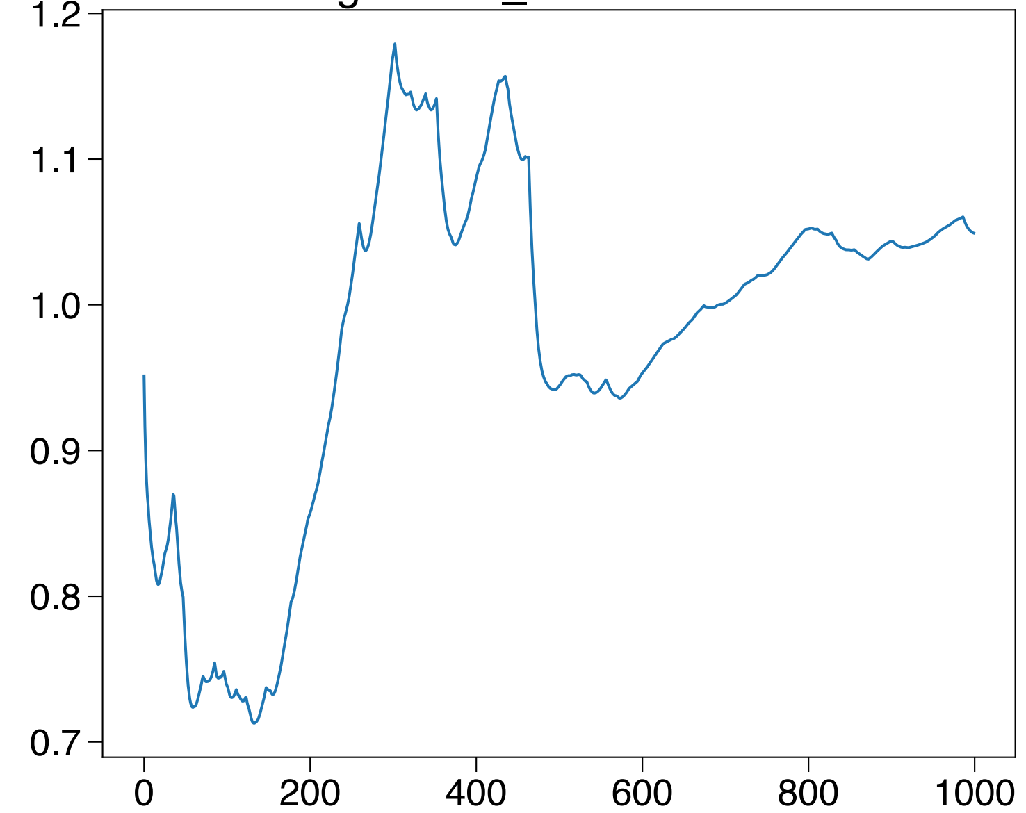
lengthscale_scale: 1.049204
