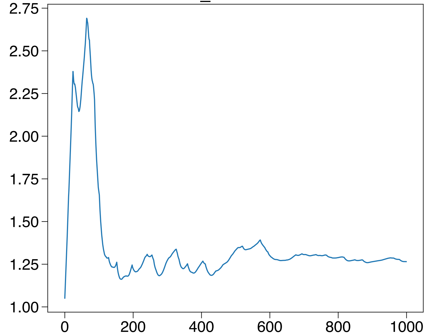
variance_scale: 1.265251
