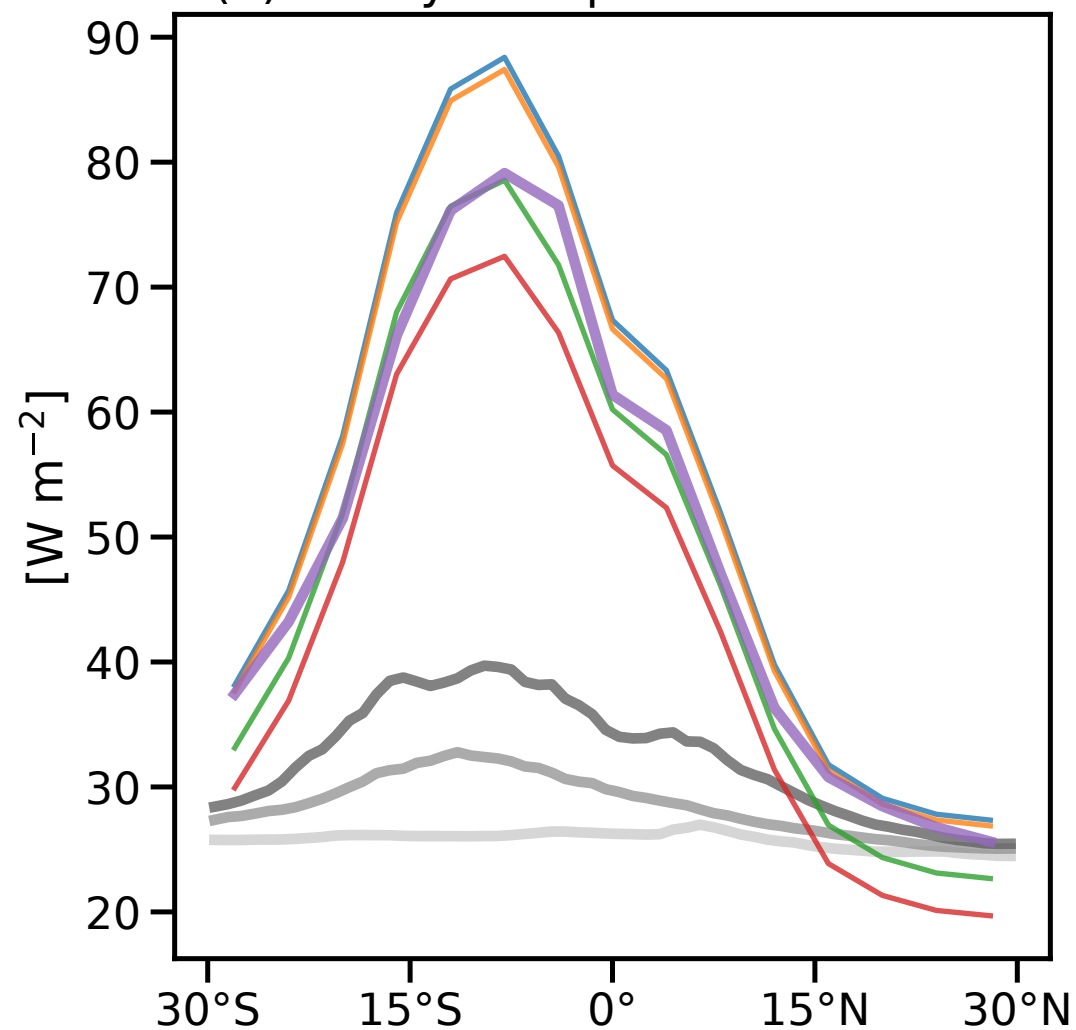
(d) all-sky 200hpa downward flux
