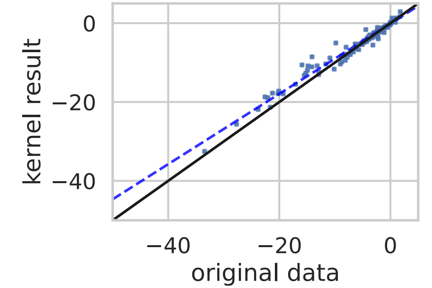
(d) ARE of SW TOA flux
