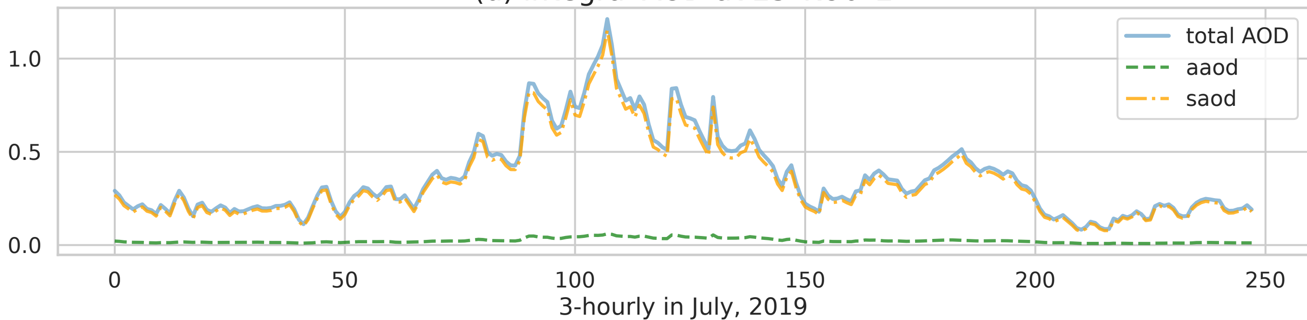
(d) integral AOD at 25°N90°E
