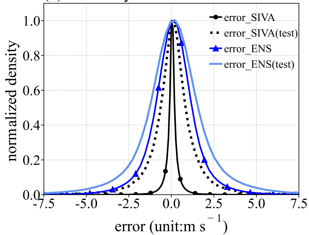
(d) U analysis errors in summer
