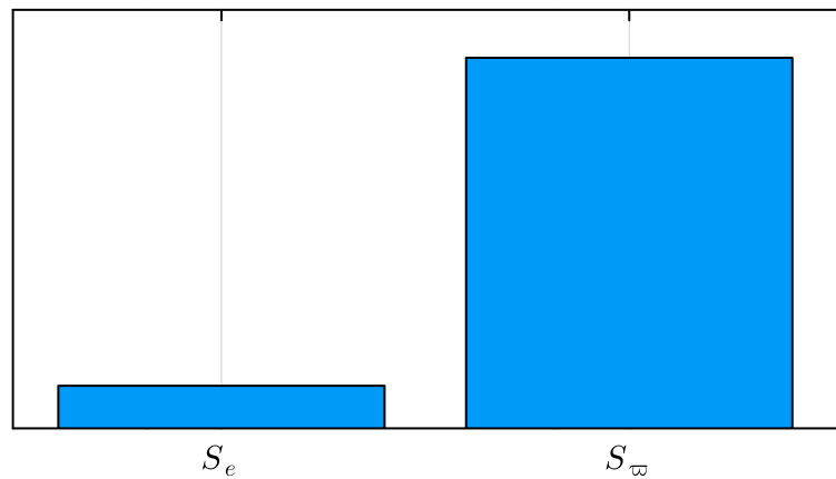
(d) \lambda_4/\lambda_{\text{tot}} = 0.0031
