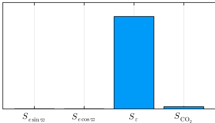
(d) \lambda_4/\lambda_{\text{tot}} = 0.0031
