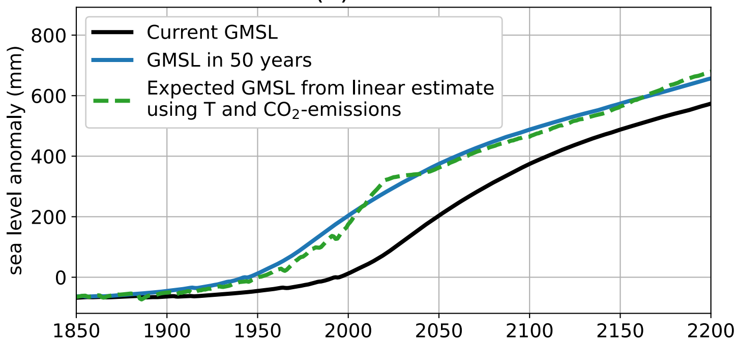
(a) SSP1-1.9
