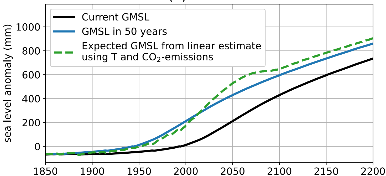
(b) SSP2-4.5
