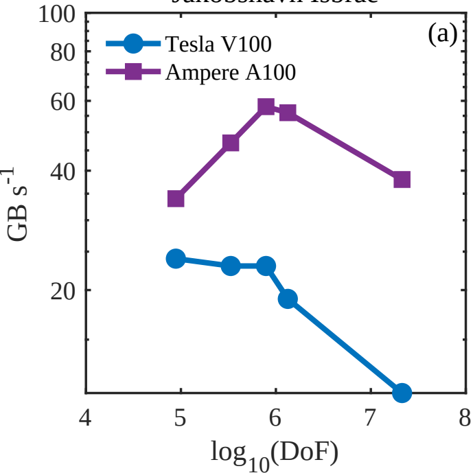
Jakobshavn Isbrae
