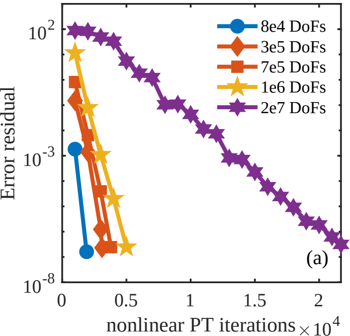
Jakobshavan Isbrae
