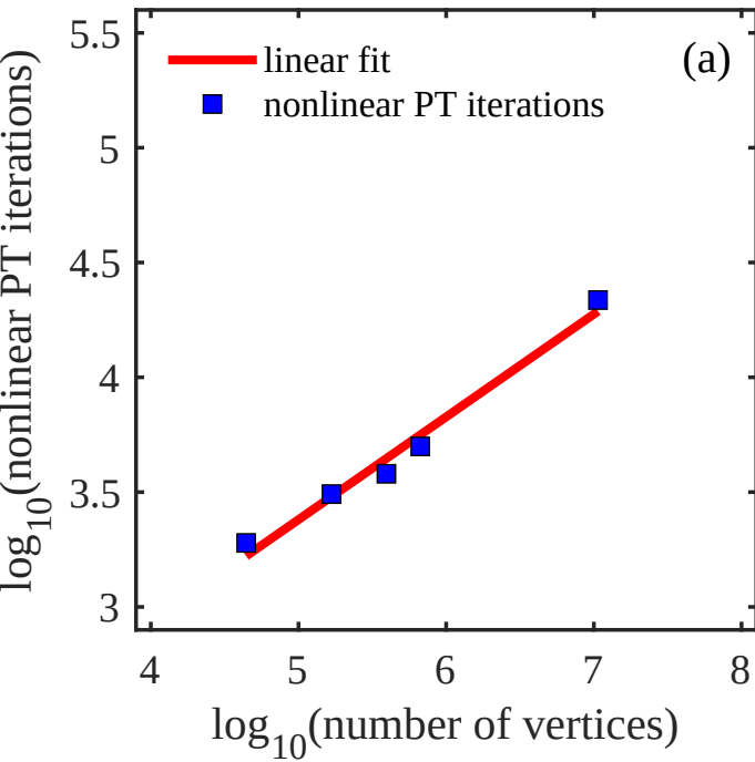
Jakobshavan Isbrae
