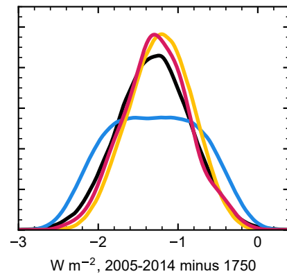
Aerosol ERF
