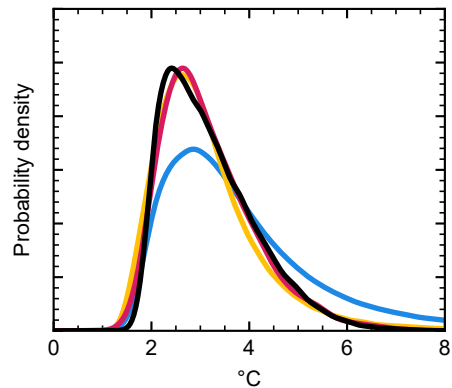
Aerosol ERFari
