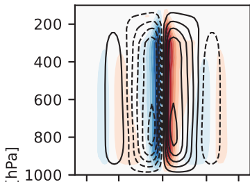
(c) CESM2
