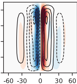
(d) Isca
