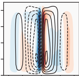
(b) CESM1
