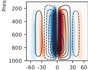
(c) CESM2
